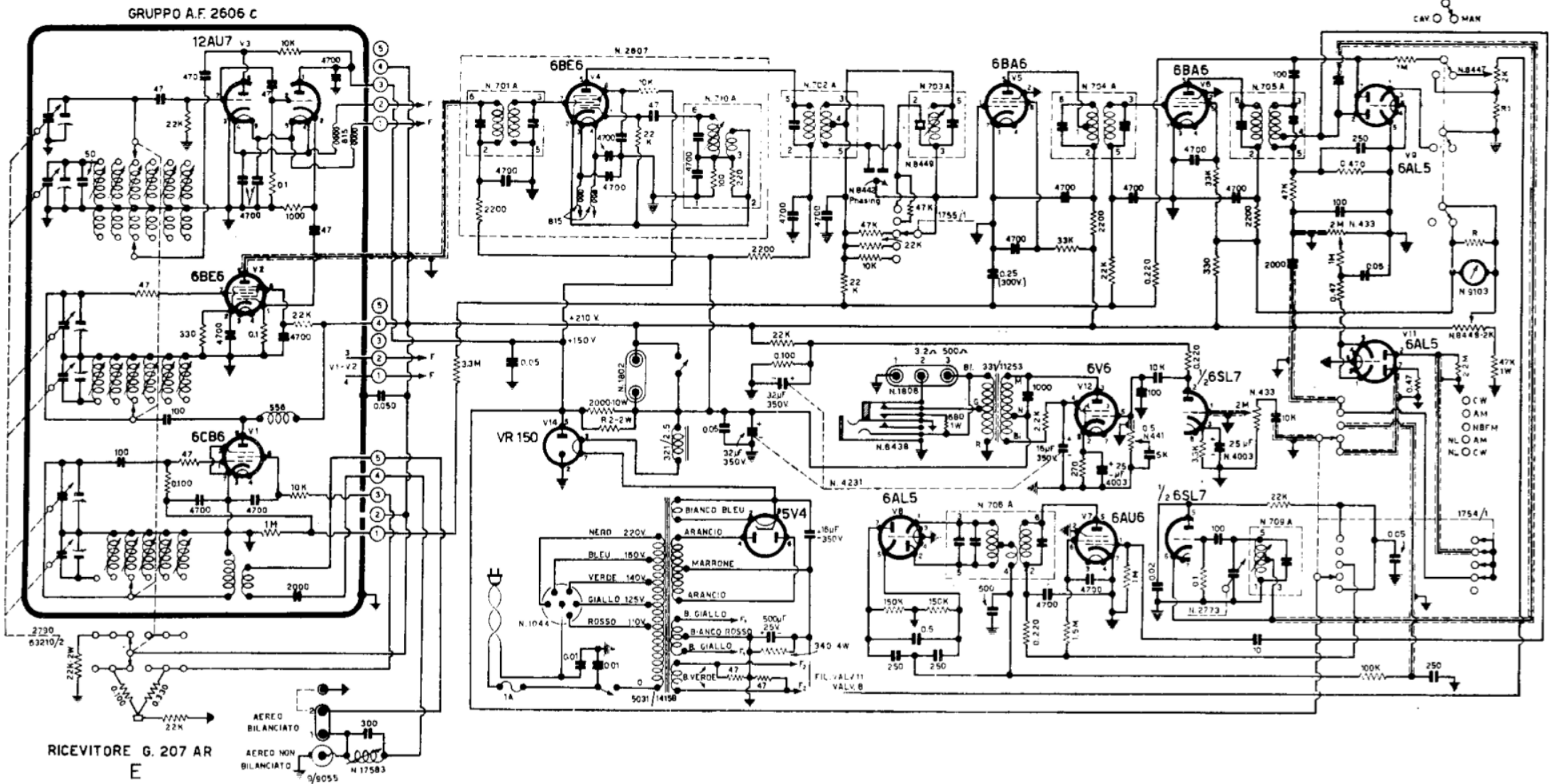
LO SCHEMA ELETTRICO DEL RICEVITORE PER ONDE CORTE G.207-AR
